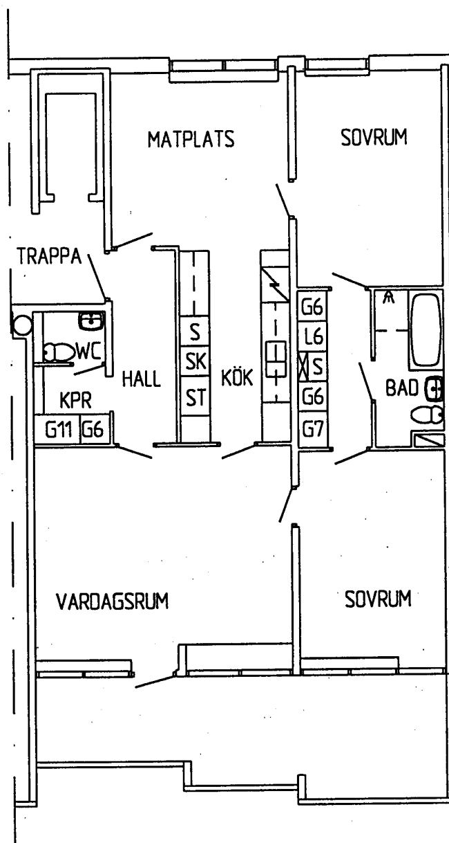
PLAN LÄGENHET, 3 ROK, CA. 90 KVM -1:100-
